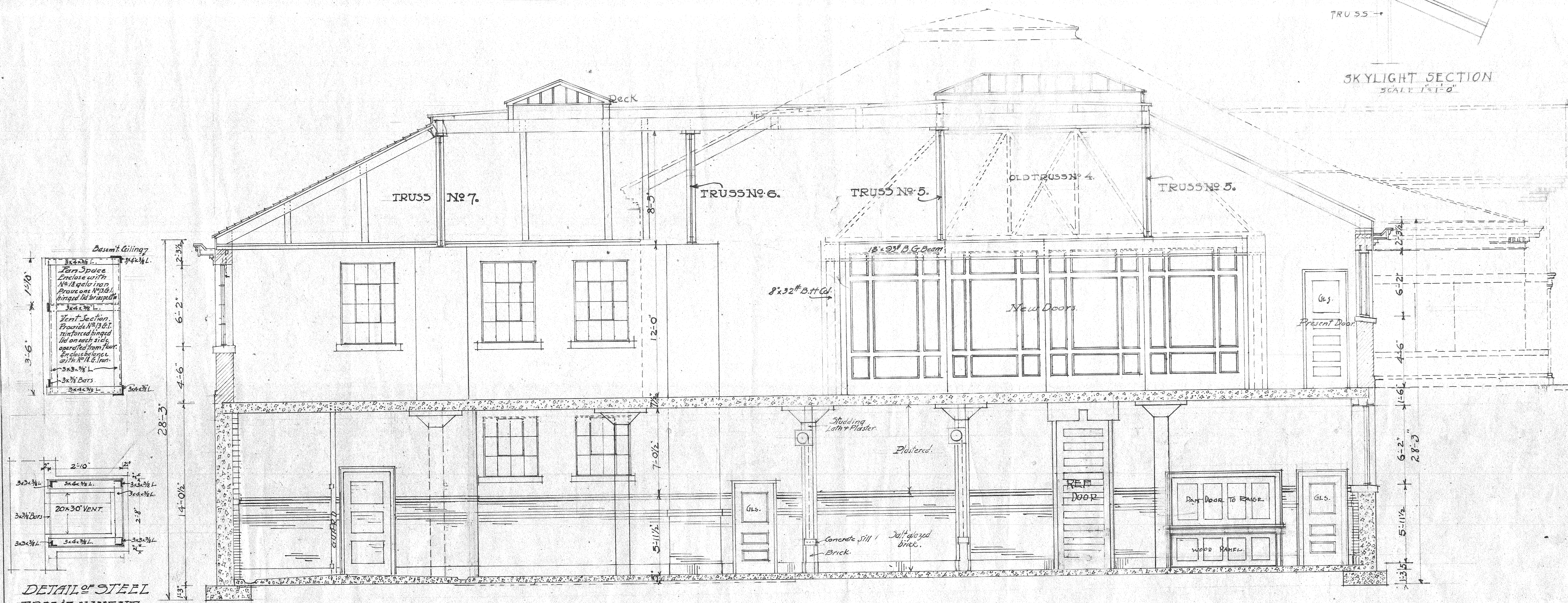
LONGITUDINAL SECTION.
